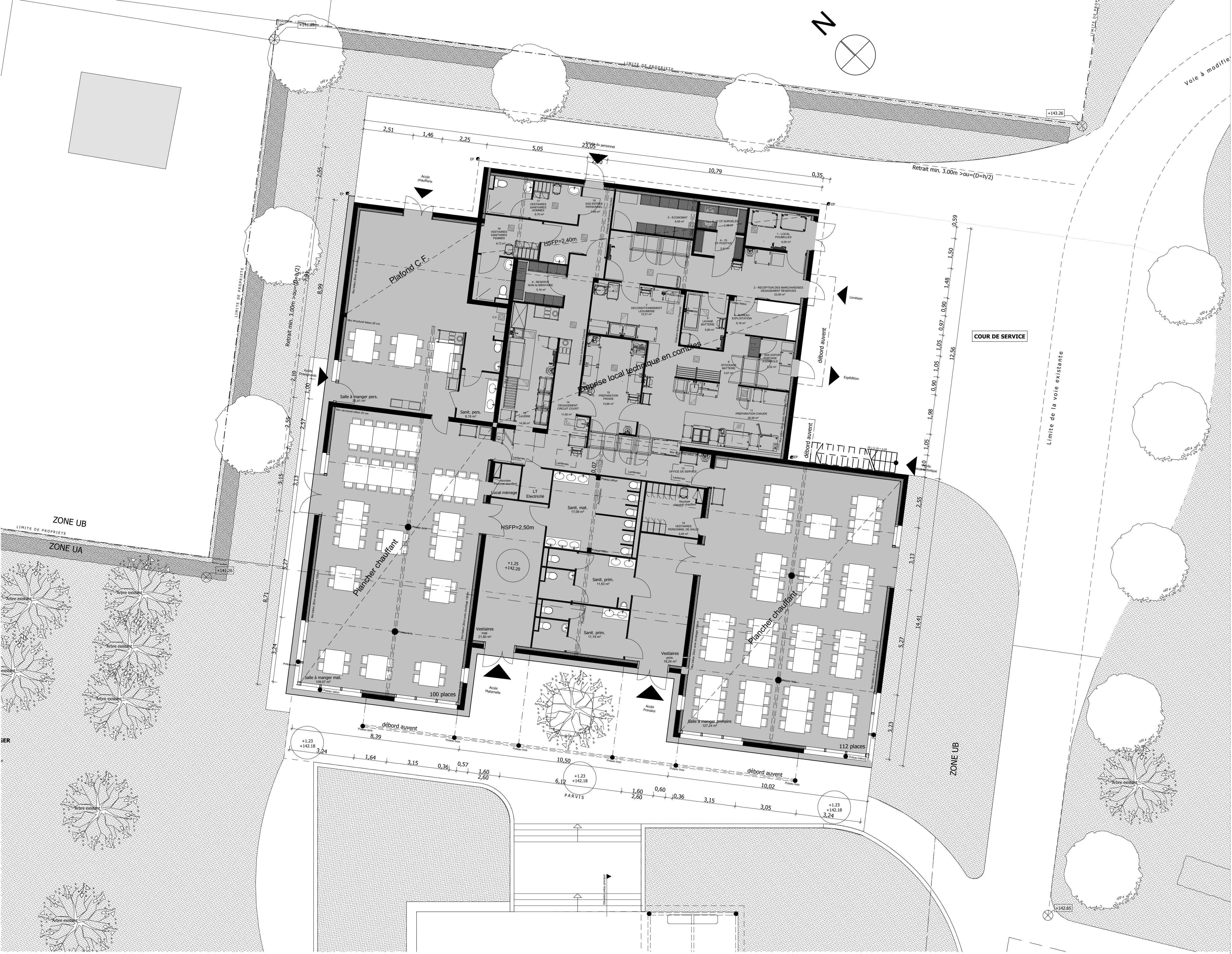
Rez-de-chaussée 1:100 1:100
